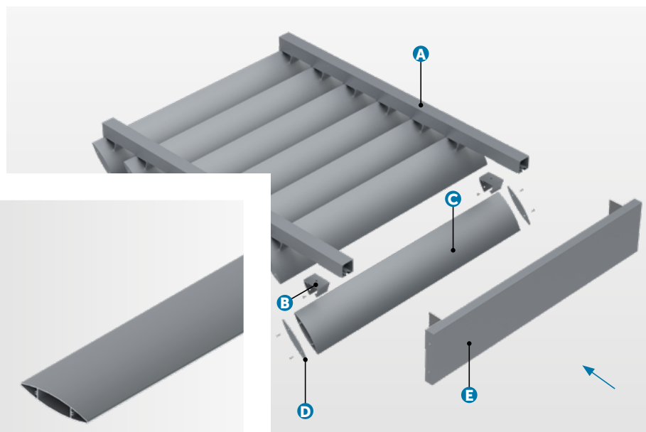
POSE HORIZONTALE PAR SPEED FIX
