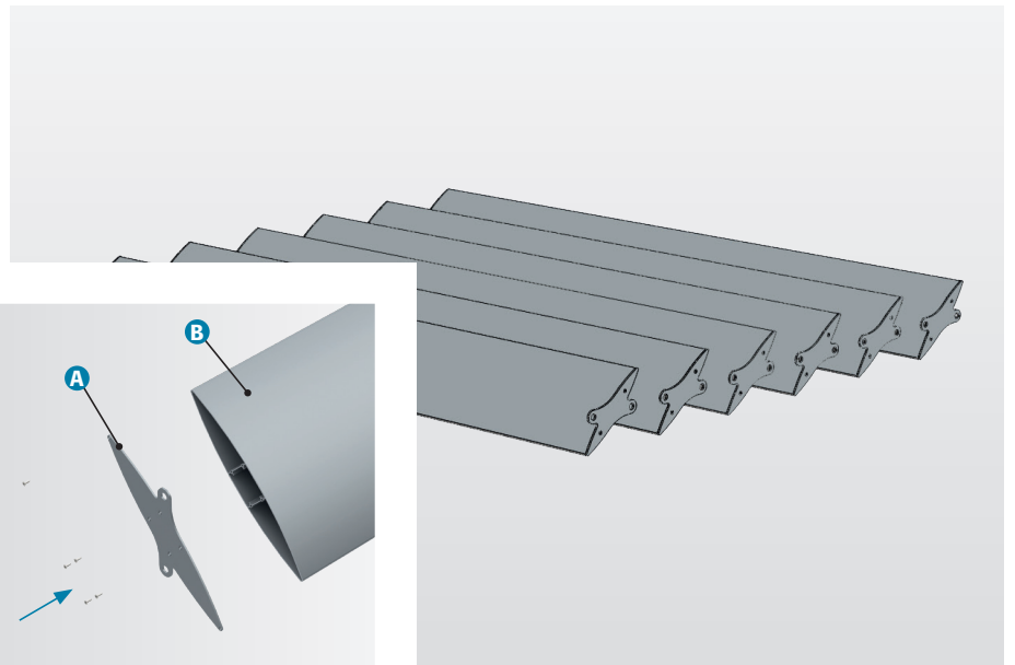
POSE HORIZONTALE | ENTRE EMBOUTS À OREILLES
