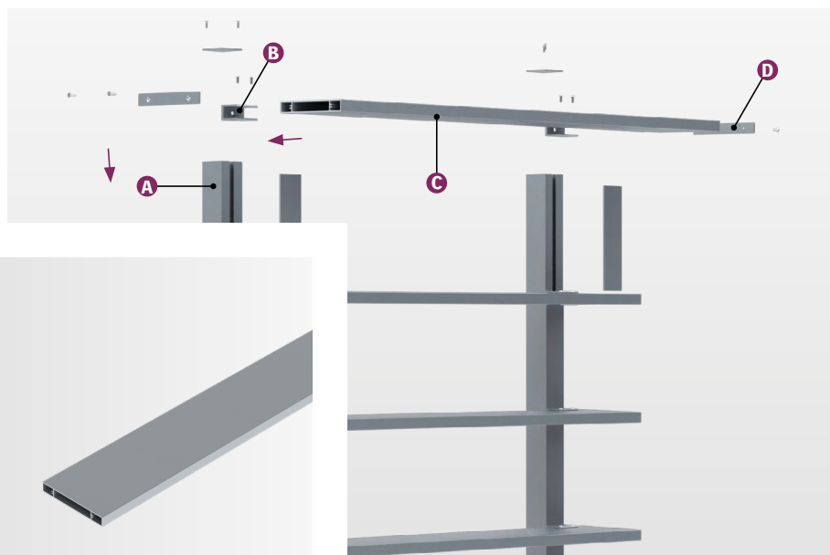
POSE VERTICALE LAMES COUCHÉES PAR FOURCHETTES SPEEDFIX
